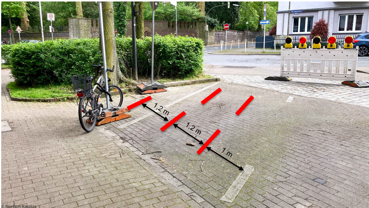
Bild 2 mit Kennzeichnung für 5 Fahrradbügel
